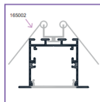
① Colocar las grapas y los conectores de perfiles
