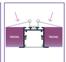
③ Dejar caer las aletas de las grapas al empotrarlo y encajar el perfil
